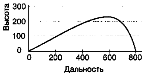
Рис. КП.3 Движение тела под углом 30° с начальной скоростью 600 м/с
