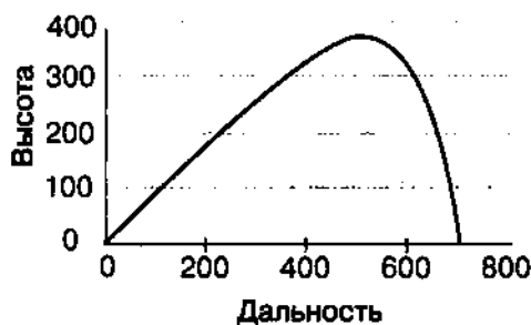
Рис. КП.2 Движение тела под углом 45° с начальной скоростью 600 м/с
